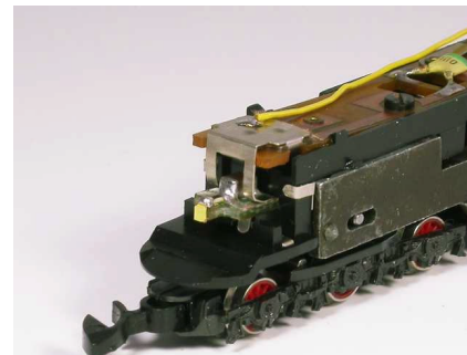
Bild 4: So sieht es dann fertig aus: Baustein ist eingesetzt. Nicht sichtbar, die richtige Polarität der unten liegenden Diodenplättchen.
