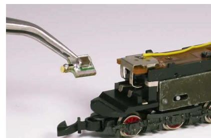
Bild 3: Richtiges Einsetzen des Bausteines – erfolgt im Prinzip wie beim analogen Einbau.
