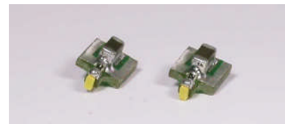
Bild 1: die gleichen Bausteine für eine digitalisierte E-Lok. Man kann die Gleichheit der Bausteine nur noch an den gleich angeordneten Diodenringen an der Unterseite sehen. Die Kondensatoren sind hier ohne Polarität. Form und Farbe der Kondensatoren und der Platine können von Baustein zu Baustein variieren.
